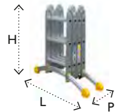
Escalera plegada: dimensiones mínimas (LxHxP) - MPA 320 : 885x925x280mm - MPA 420 : 885x1175x280mm
